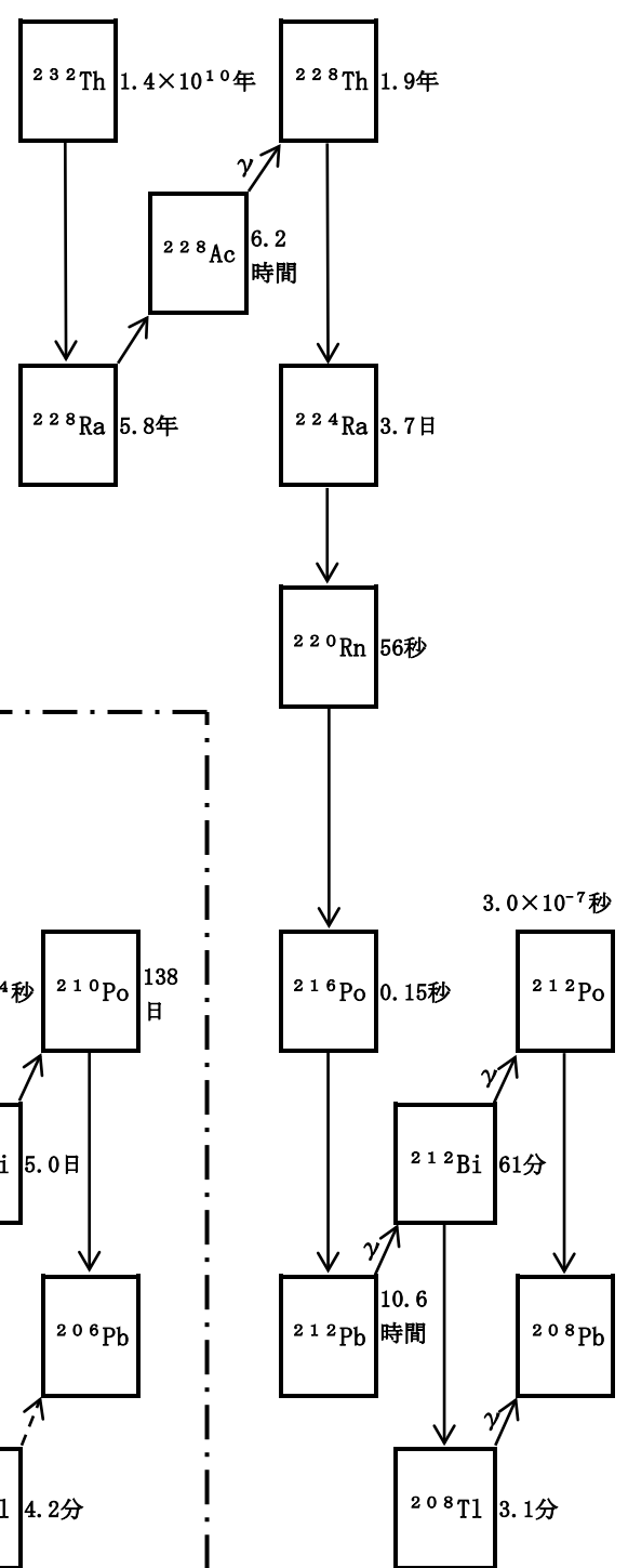
図 II - 2 トリウム系列
