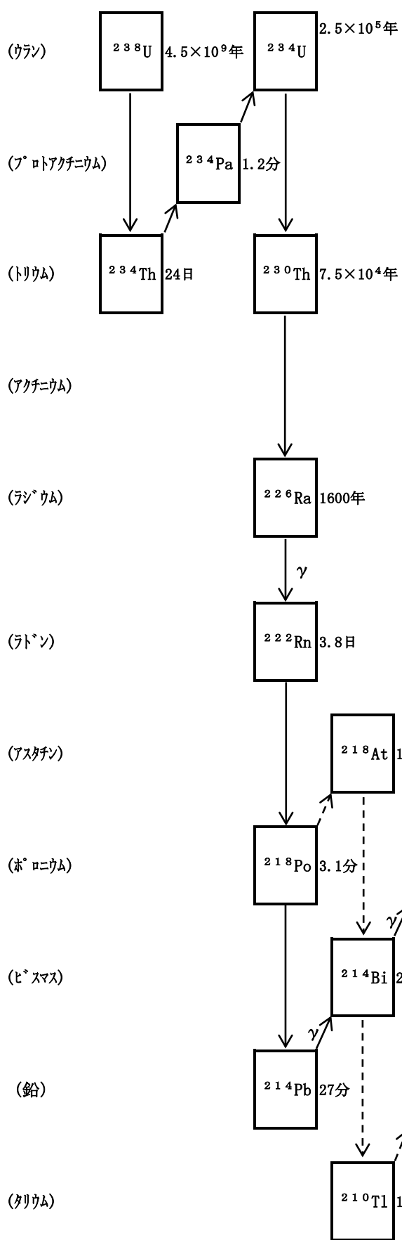
図 II - 1 ウラン系列
